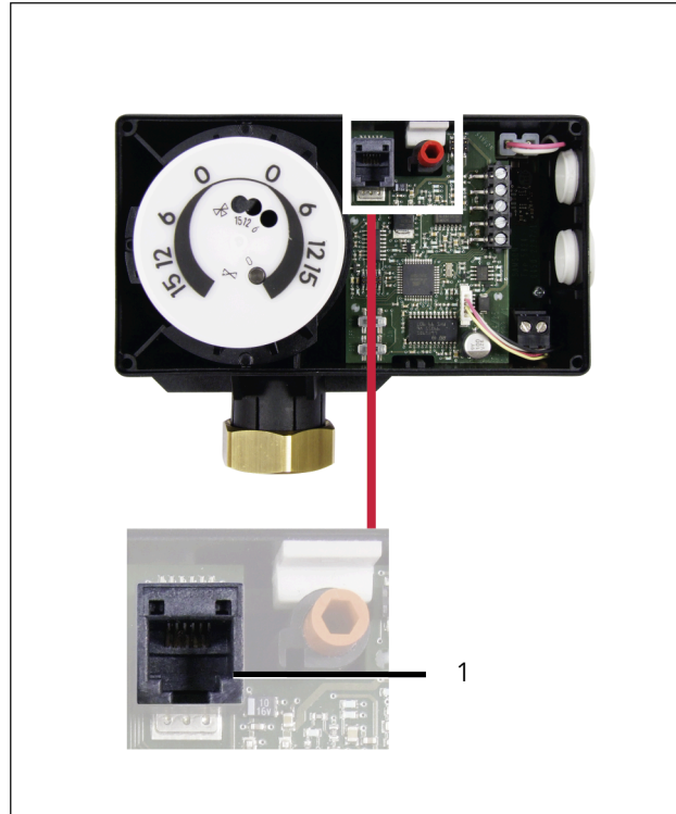
Bild 2: Serielle Schnittstelle
