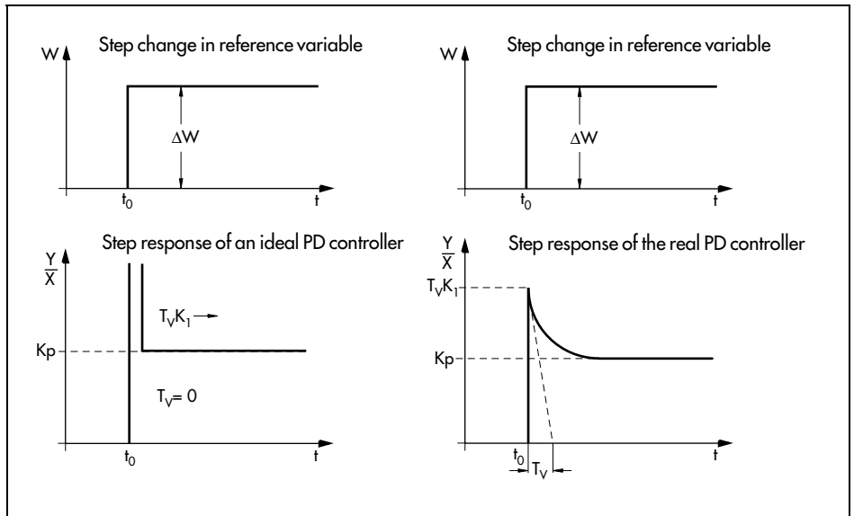
Fig. 62 · PD controller
