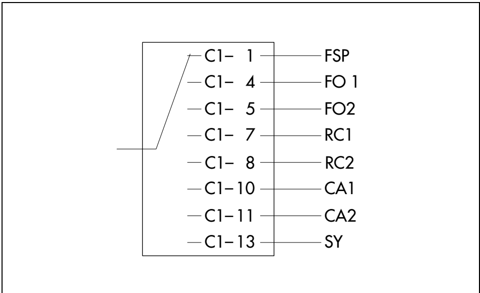
Fig. 22 · Control modes
