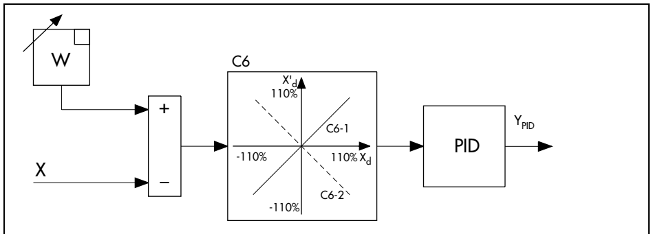
Fig. 48 · Inversion of error
