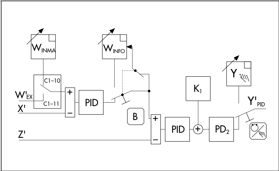
Fig. 26 · Cascade control
