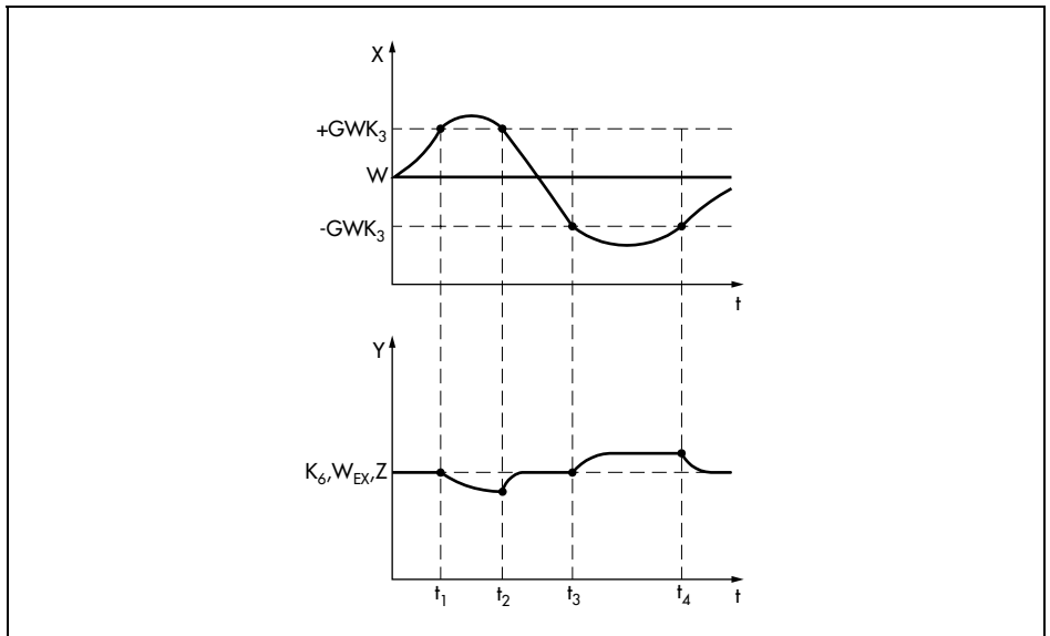
Fig. 71 · Y_0/PI(D) change of control action
