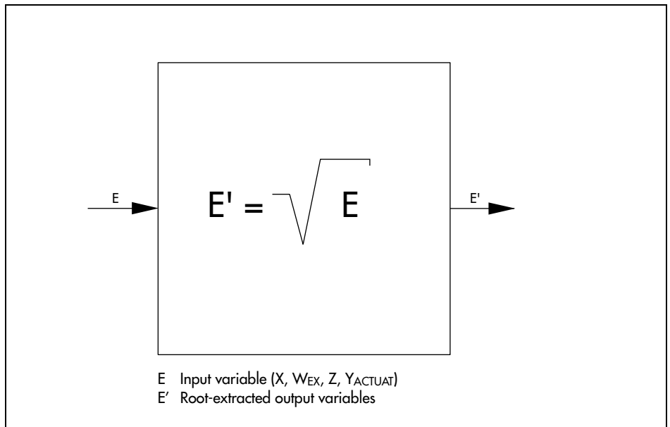
Fig. 4 · Root-extraction
