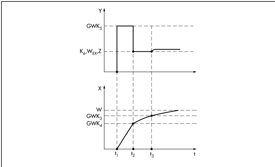
Fig. 72 · Y_{\max}/Y_0/PI(D) change of control action
