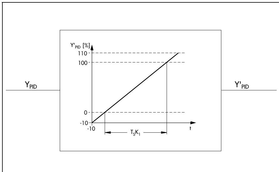
Fig. 56 · Output ramp
