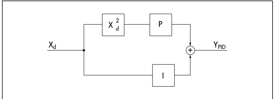
Fig. 64 · P 2 I controller
