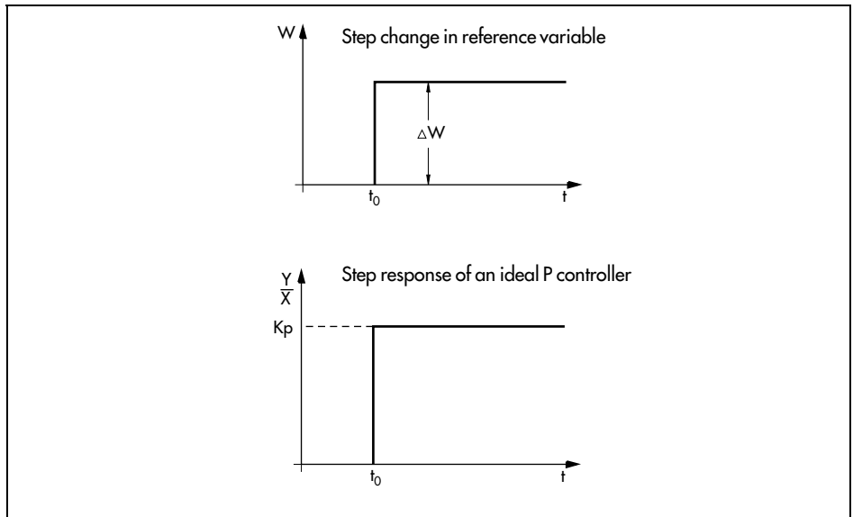
Fig. 60 · P controller
