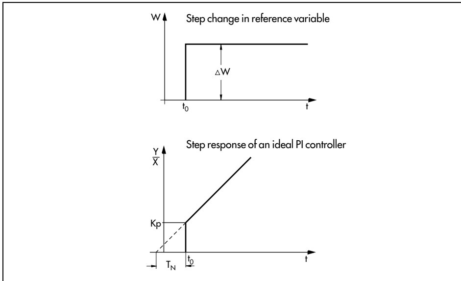
Fig. 61 · PI controller
