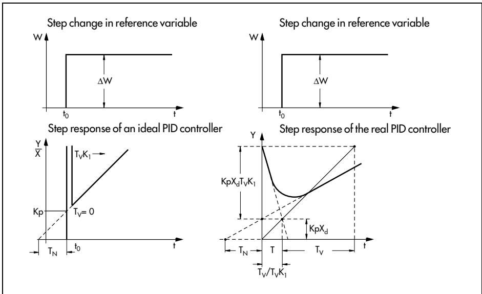
Fig. 63 · PID controller
