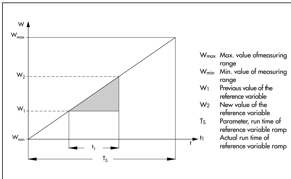
Fig. 53 · Reference variable ramp
