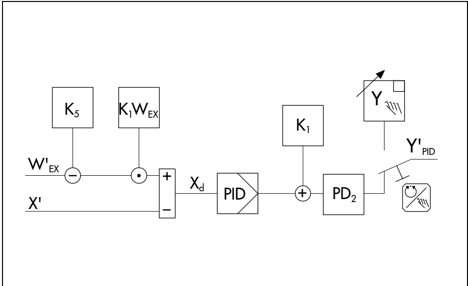
Fig. 30 · Synchro control
