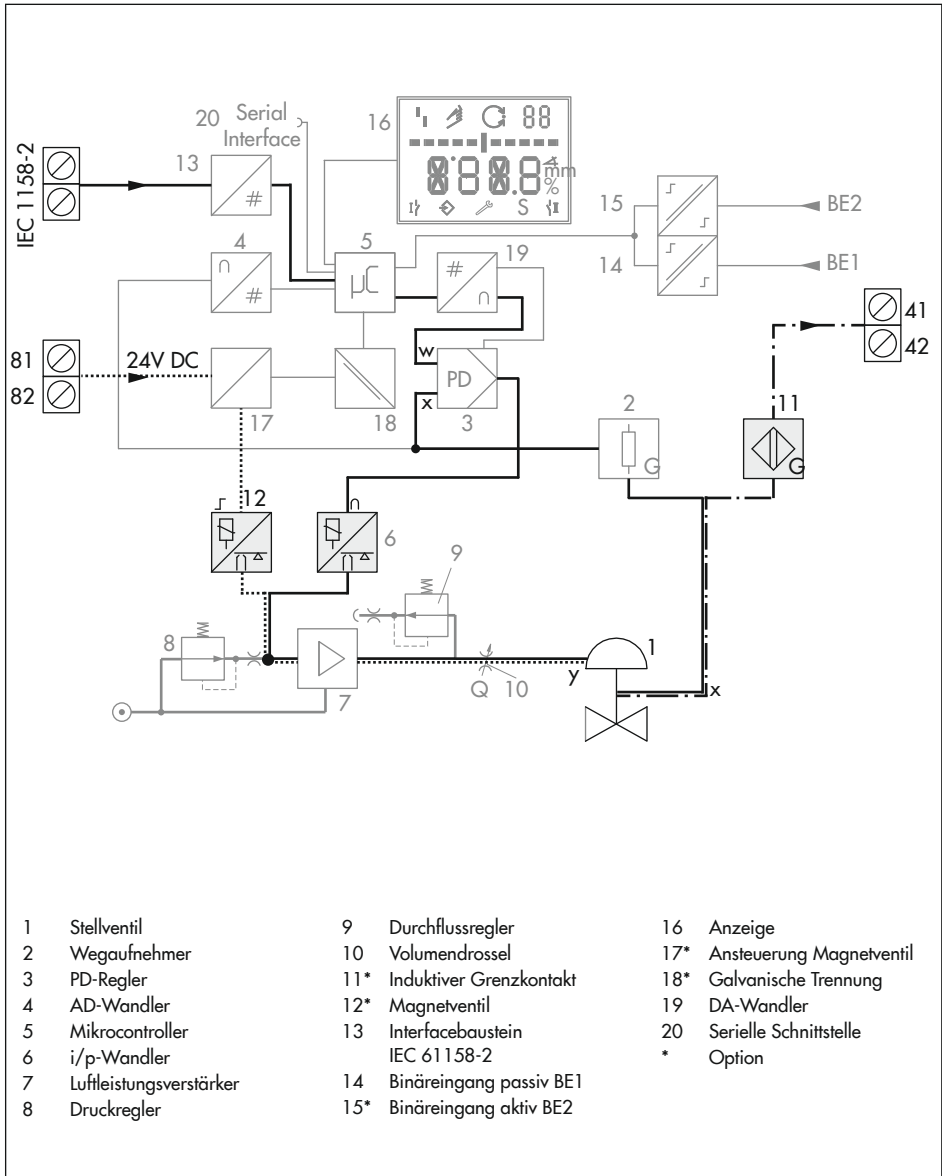
Bild 1: Wirkungsweise des Stellungsreglers
